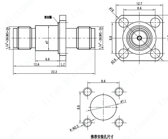
推荐安装孔尺寸
